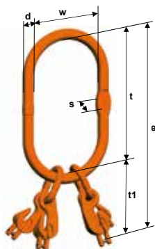
LXKW 4 Kuppelaufhängegarnitur
