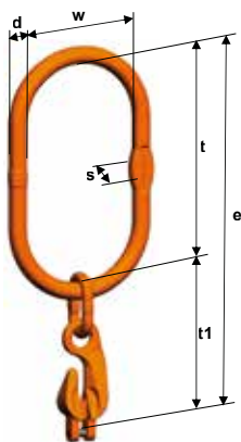
LXKW 1 Kuppelaufhängegarnitur
