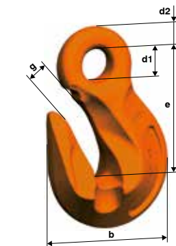
Form mit Stützfläche
