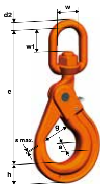
WLHW Wirbelsicherheitslasthaken
