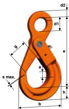
LHW Sicherheitslasthaken
