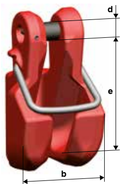
KVS Kuppelverbinder G8
