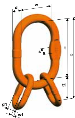
VW Vierstranggarnitur
