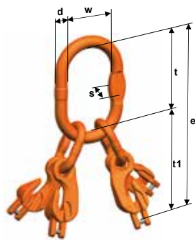
VMXKW 4 Kuppelaufhängegarnitur
