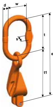
VMXKW 1 Kuppelaufhängegarnitur
