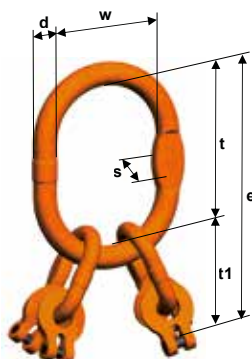
KMGW 4 Übergroße Kuppelaufhängegarnitur
