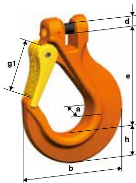
BKHSW Übergroßer Kuppelhaken
