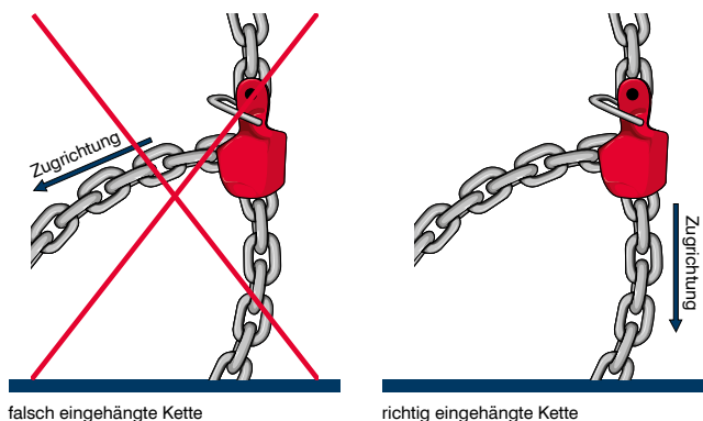
falsch eingehängte Kette
