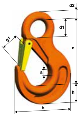
HSW Ösenhaken
