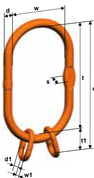
VSW 2/4 Übergroße Aufhängegarnitur
