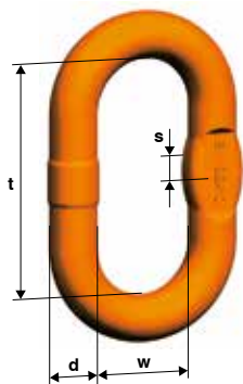
BW Übergangsglied
