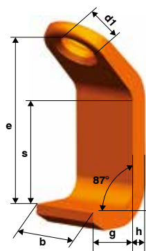
BWW Blechwinkel
