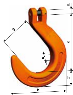
KFW Kuppelweitmaulhaken
