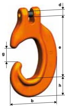
KCHW Kuppel C-Haken
