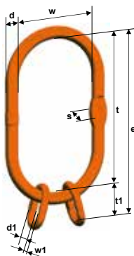
VLW 2/4 Aufhängegarnitur
